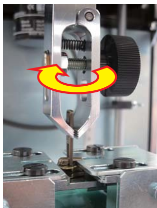
JIS S 3015 スライダー引手ねじり試験
