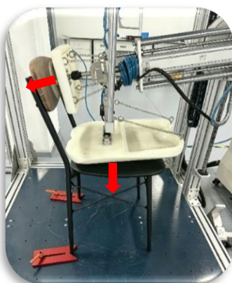
座面・背もたれの 耐久性
